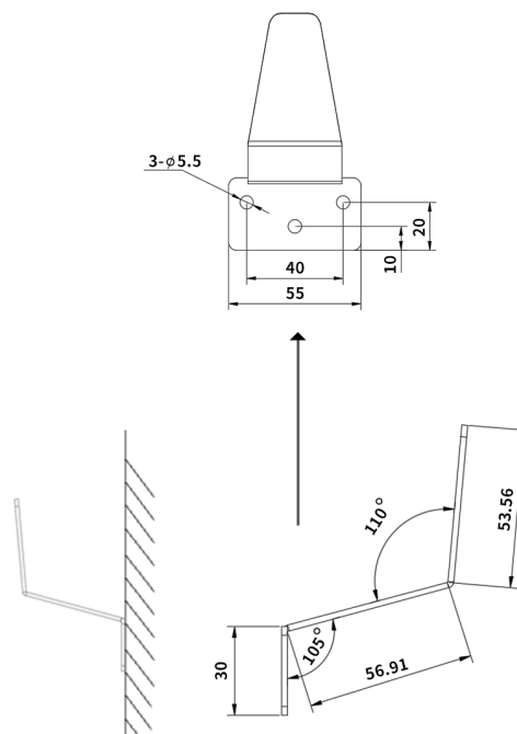
挂钩 x 1
