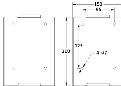
Wandplatte x 1
