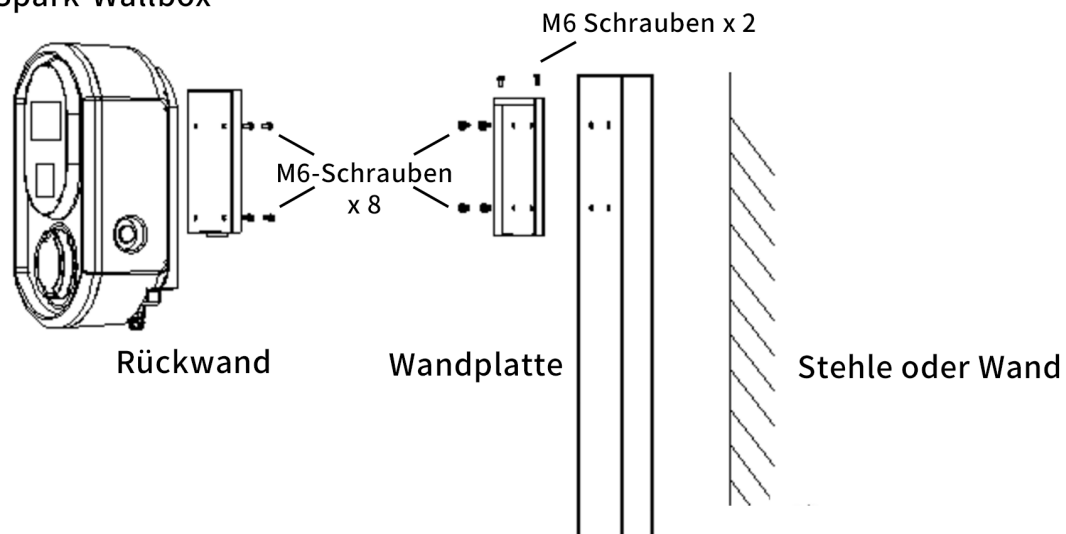
Spark-Wallbox
