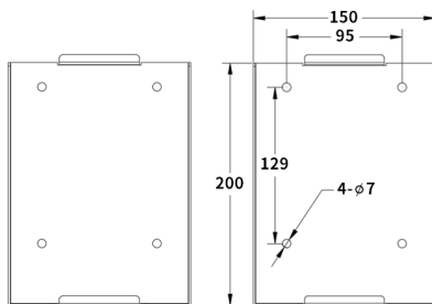
挂墙板 x 1
