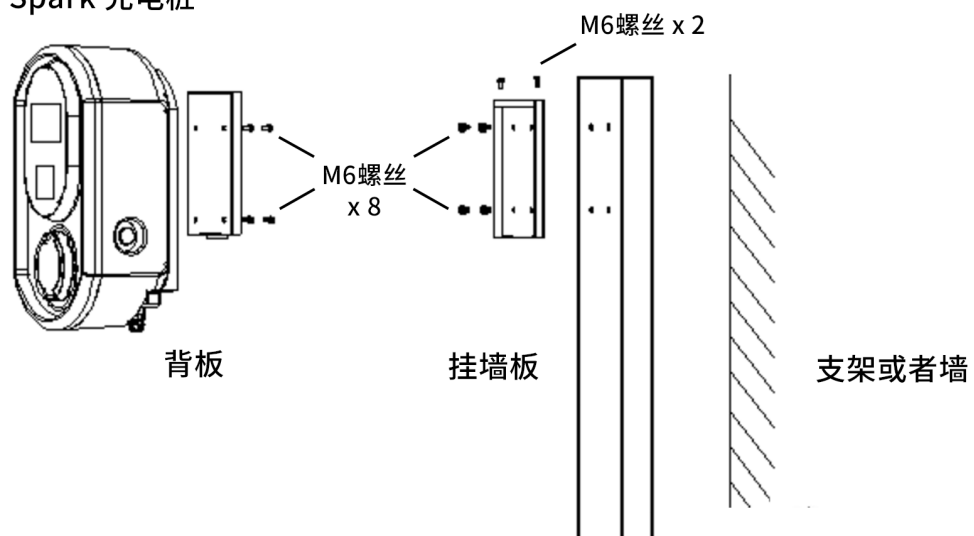
Spark 充电桩
